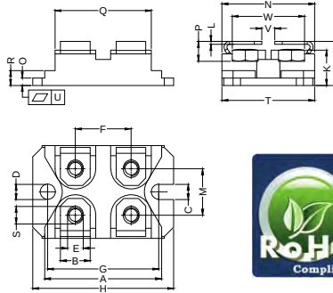
Dimensions SOT-227
