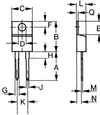
Dimensions TO-220AC
